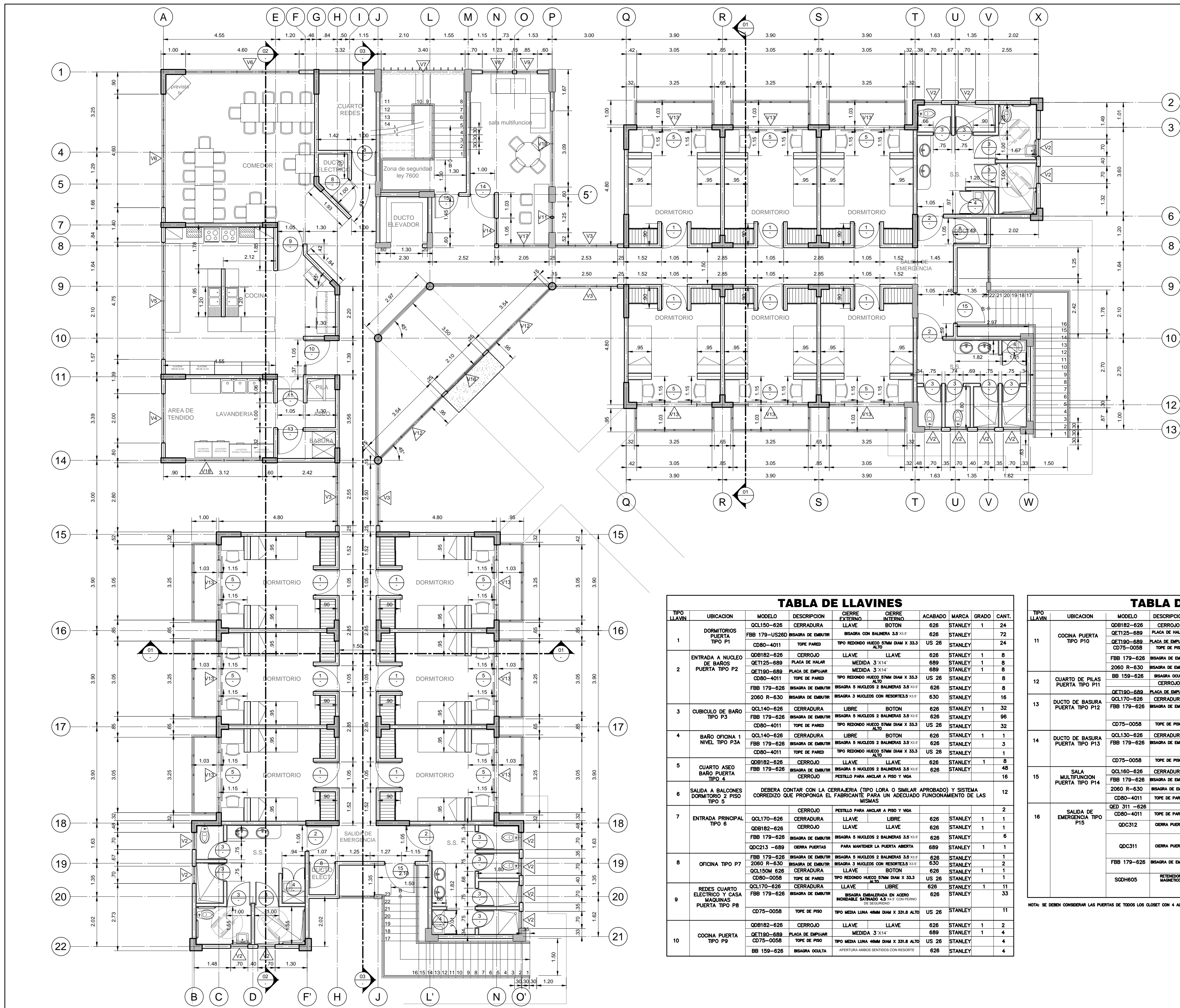
PLANTA DISTRIBUCION ARQUITECTONICA SEGUNDO NIVEL (RESIDENCIAS)
