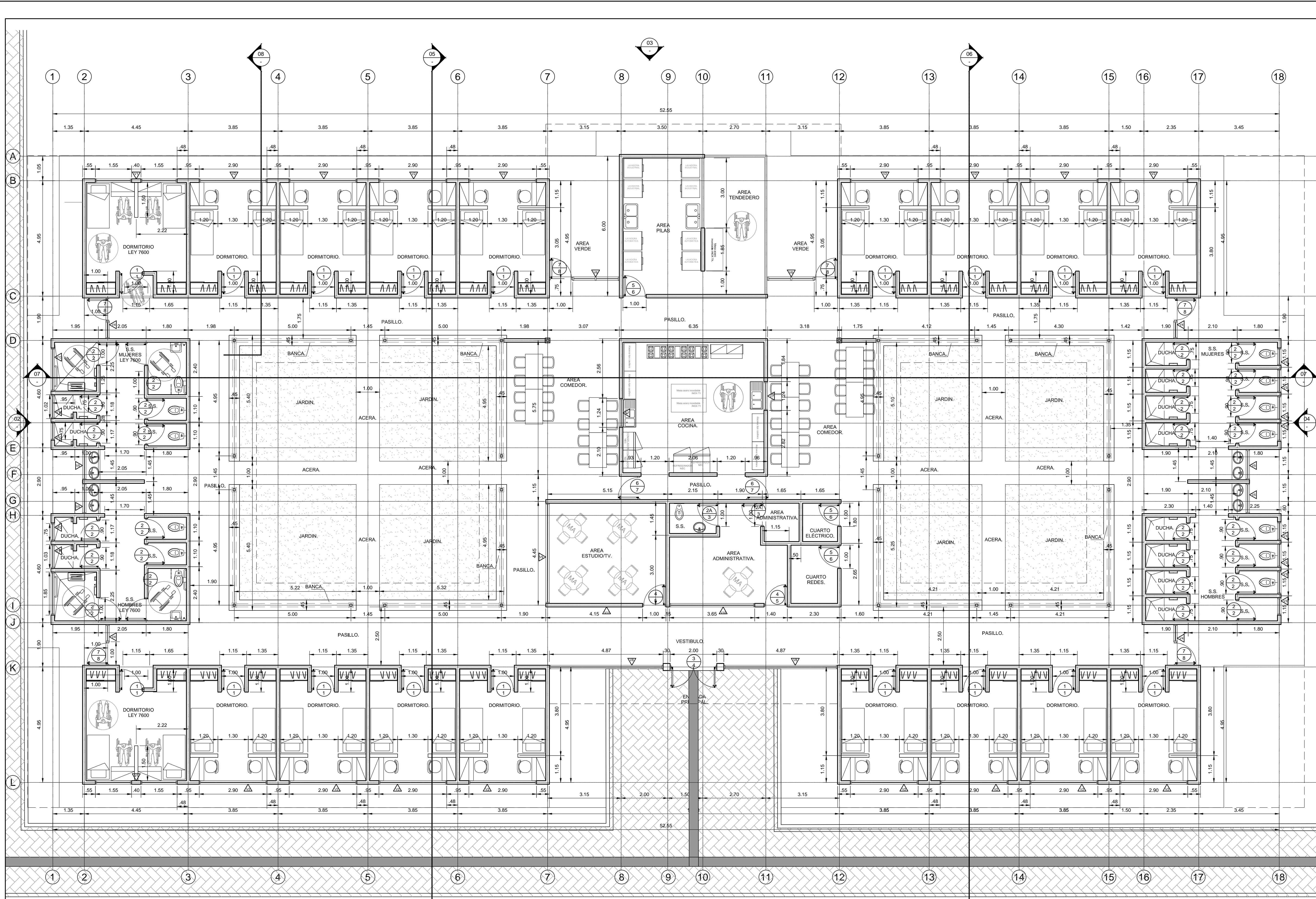
PLANTA DE DISTRIBUCION ARQUITECTONICA Y ACOTADO.
